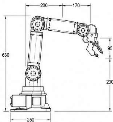
VISTA LATERAL ESCALA 1:3
